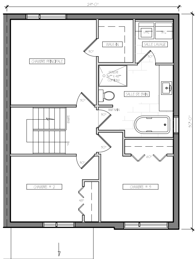
2 ÉTAGE ÉCHELLE : 1/8" = 1'-0"
