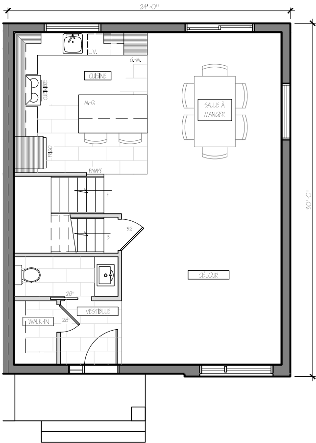
1 REZ-DE-CHAUSSÉE ÉCHELLE : 1/8" = 1'-0"
